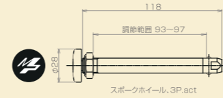
スポークホイール, 3P.act
